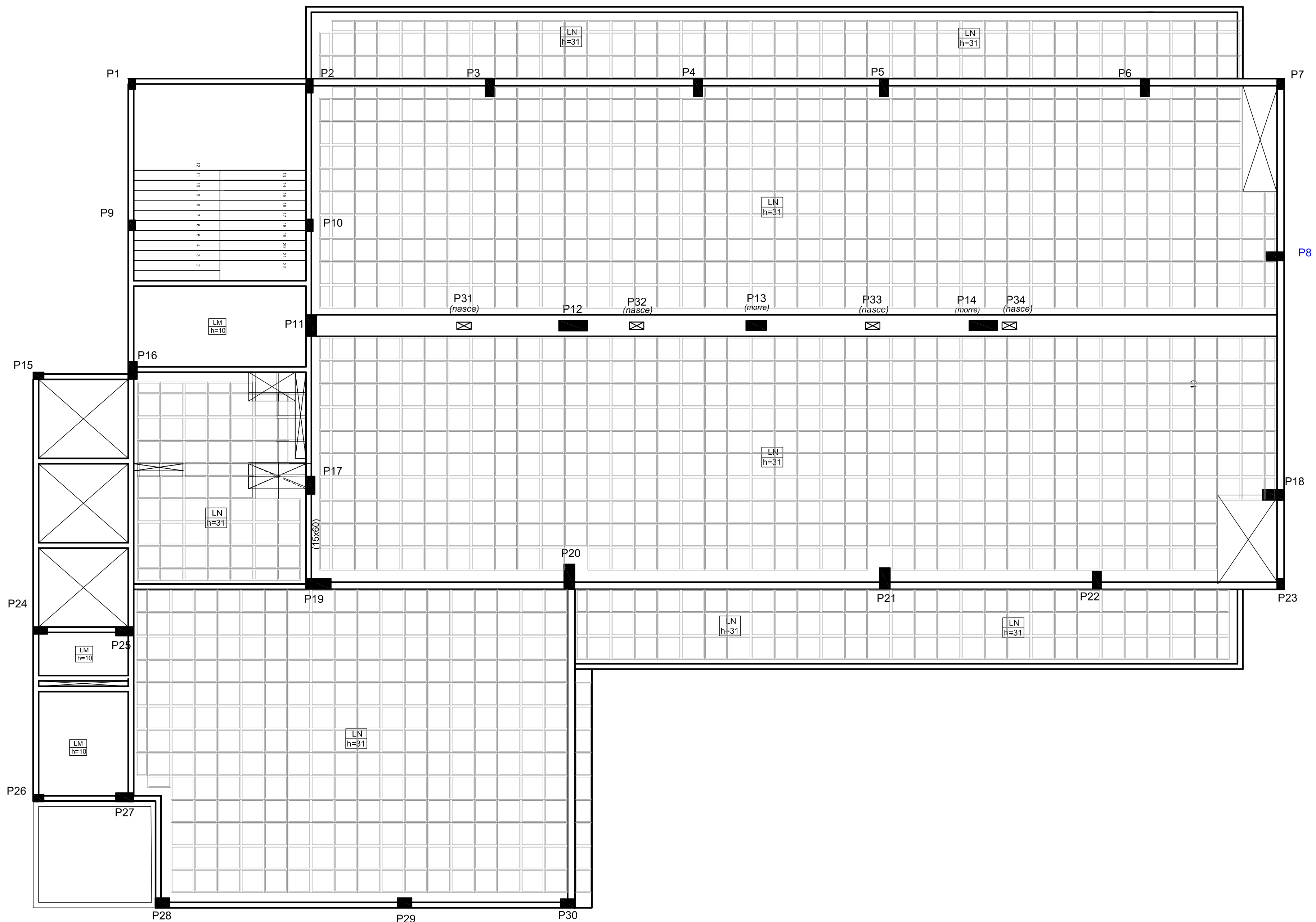
Planta de Fôrmas 4º Pavimento - Cubetas Escala 1:75
